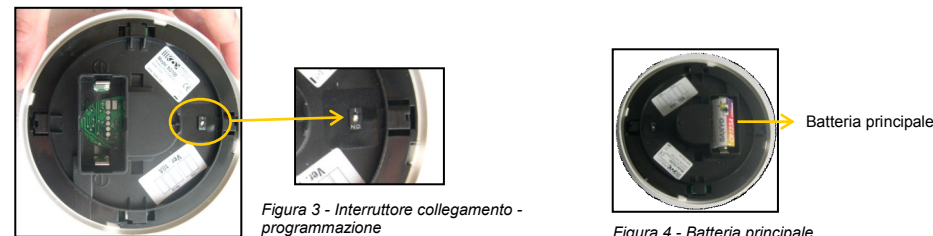
Figura 4 - Batteria principale
